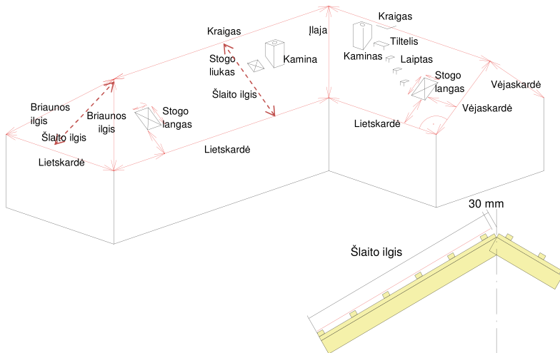
Pav. 1 - Matmenys reikalingi paskaičiuoti stogo dangai
