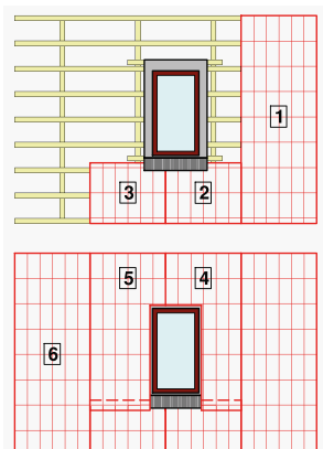
Pav. 8 – Lango ar išlipimo liuko montavimas
