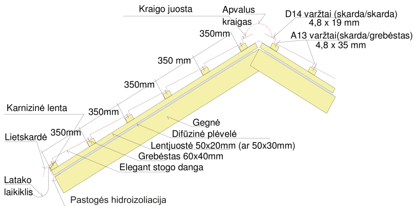
Pav. 2a - Tvirtinimas, naudojant lietskardes
