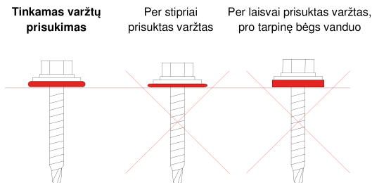
Pav. 5. - Varžtų tvirtinimo technologija
