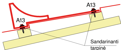
7 pav. - Sraigčių lankstinių ir priedų tvirtinimas
