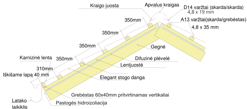
Pav. 2 b - Tvirtinimas nenaudojant lietskardžių – su 40 mm išikišusia danga
